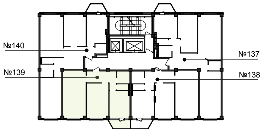
СХЕМА СЕКЦИИ №3 (3 этаж)
