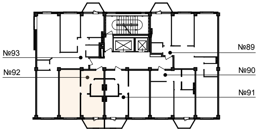
СХЕМА СЕКЦИИ №2 (3 этаж)
