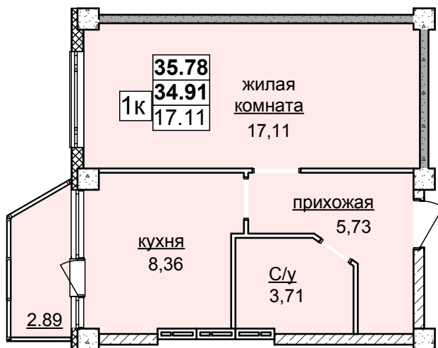
КВАРТИРА №58
